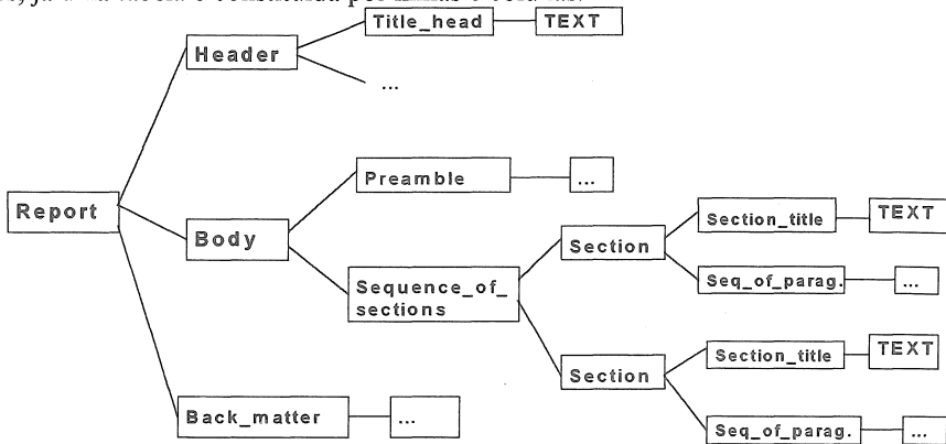
Fig 1 - Estrutura lógica de um documento [QUI 95]
